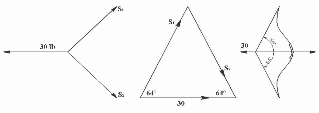
Şekil 1: 30 lb'lik bir çekiş ağırlığında kirişe uygulanan yük miktarı.
