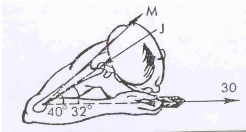
Şekil 3: Kolu horizontal abdüksiyonda tutmak için gerekli kas kuvvetinin analizi. M: Deltoid kasının arka huzmeleri, J: Glenohumeral eklemdeki güç.
